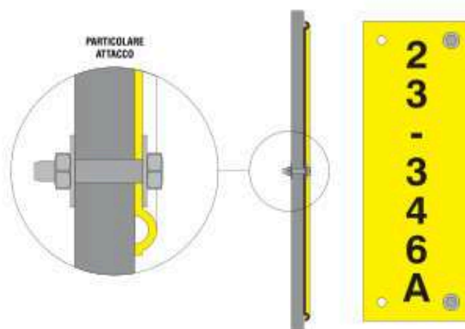
D TARGA CON NUMERO DI TERNA
